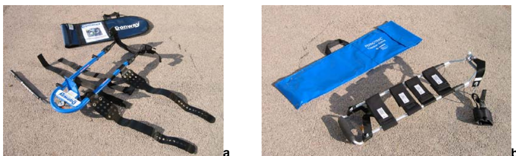
Figure 8.28 : Attelles en traction pneumatique (a) et manuelle (b)
